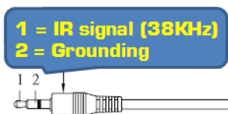
IR Blaster
